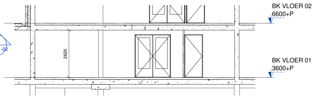
Doorsnede 02
