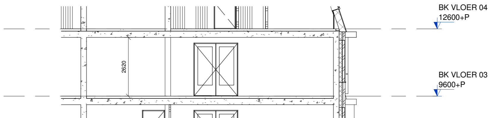
Doorsnede 13
