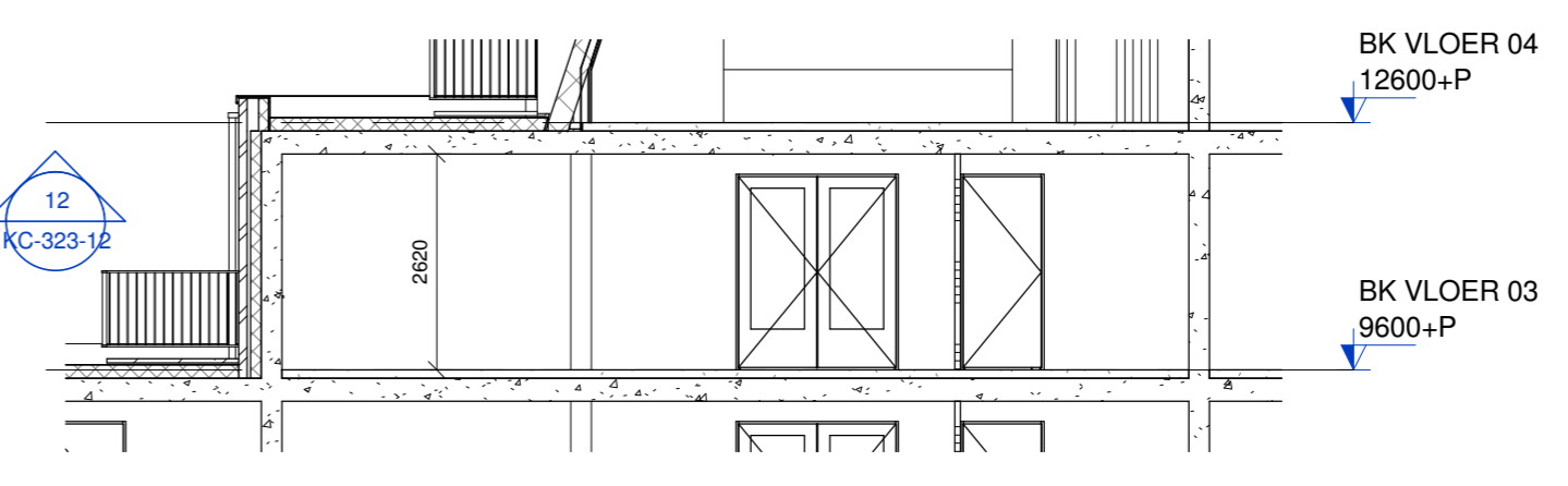
Doorsnede 12
